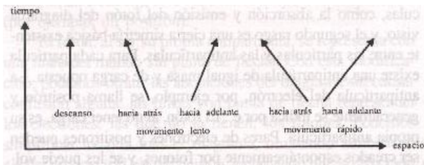
Líneas del mundo de partículas
